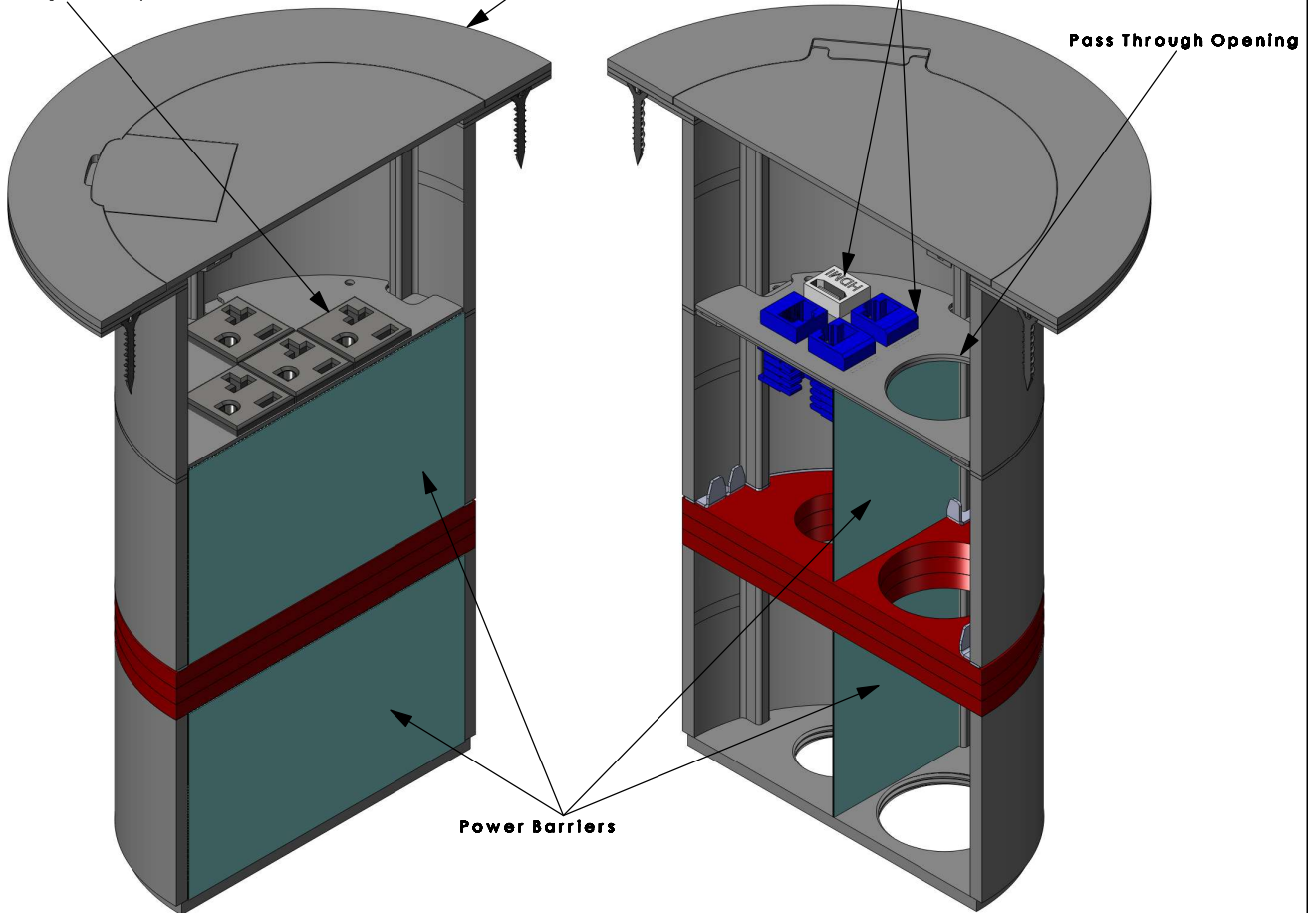
15A or 20A Single Receptacles
