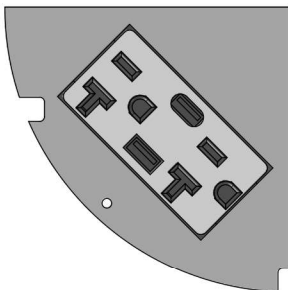
Decora Connector Plate (* 15A or 20A, Usb Type A/Type C Receptacles)
